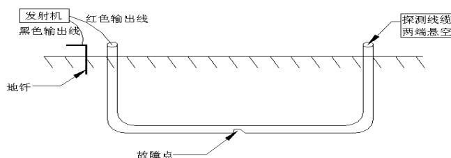
图 1 发射机连接图
