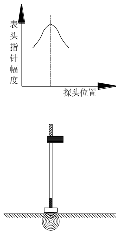
图 2 峰值法
