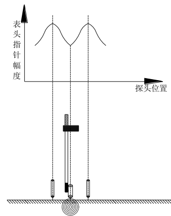
图 3 空值法
